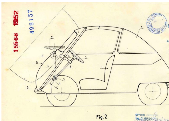
Isetta, 1953
